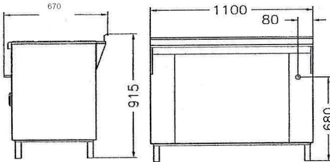
DIMENSIONES MAXIMAS
